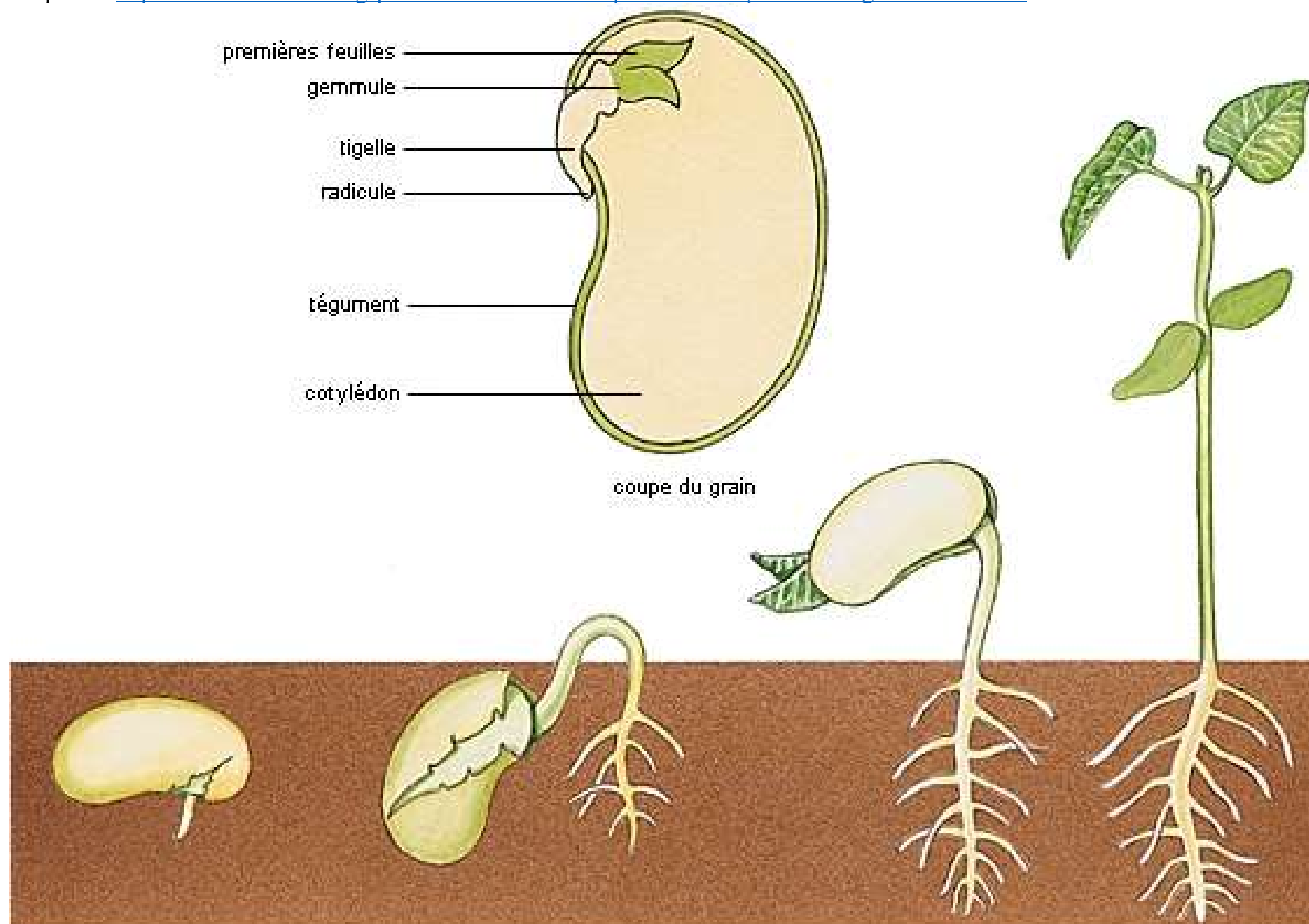
Coupe de la graine et phases de la germination épigée du haricot (les cotylédons sont soulevés au-dessus du sol).
